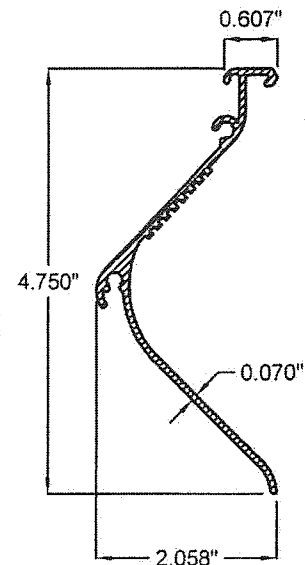
5 BLADE
