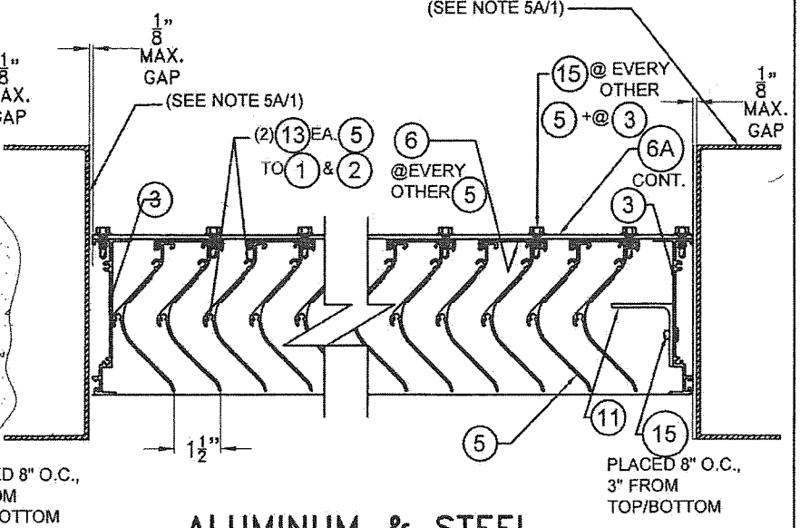
ALUMINUM & STEEL SUBSTRATE N.T.S.
