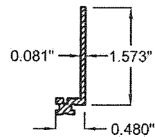
9 FLANGE
