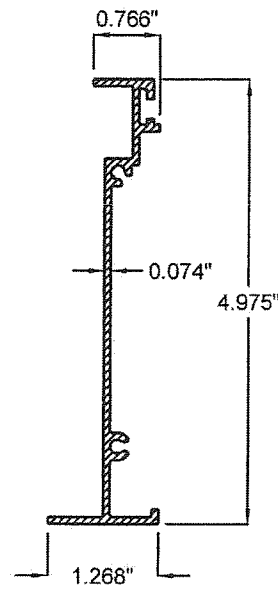
3 SIDE JAMB
